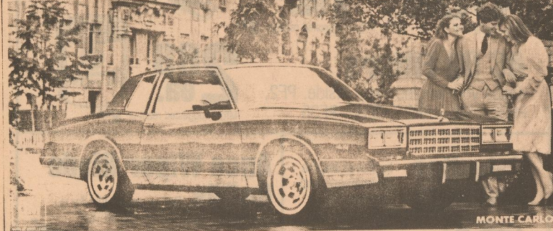
MONTE CARLO
